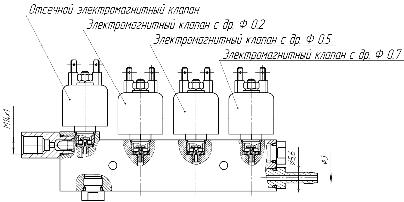
Рис. 3- Блок низкого давления
