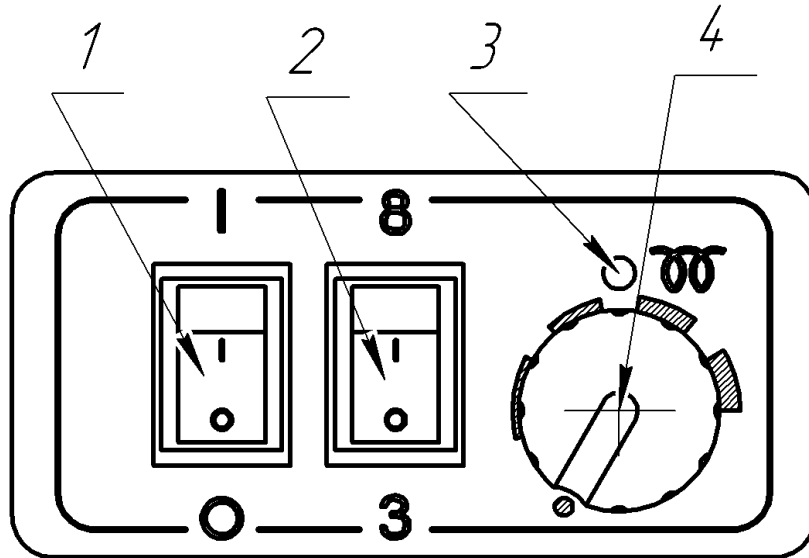
Рис. 5 – Лицевая панель пульта управления
